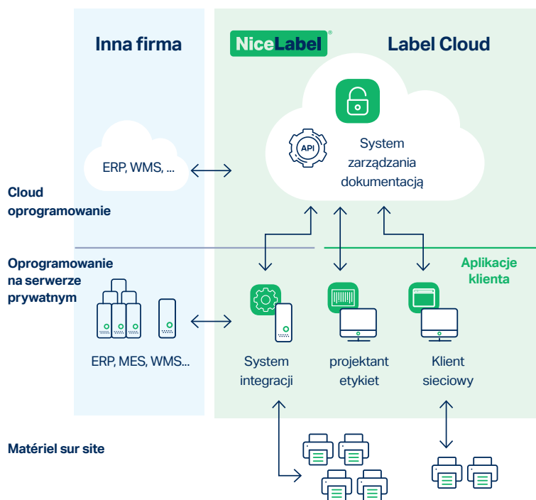
Architektura systemu Label Cloud
